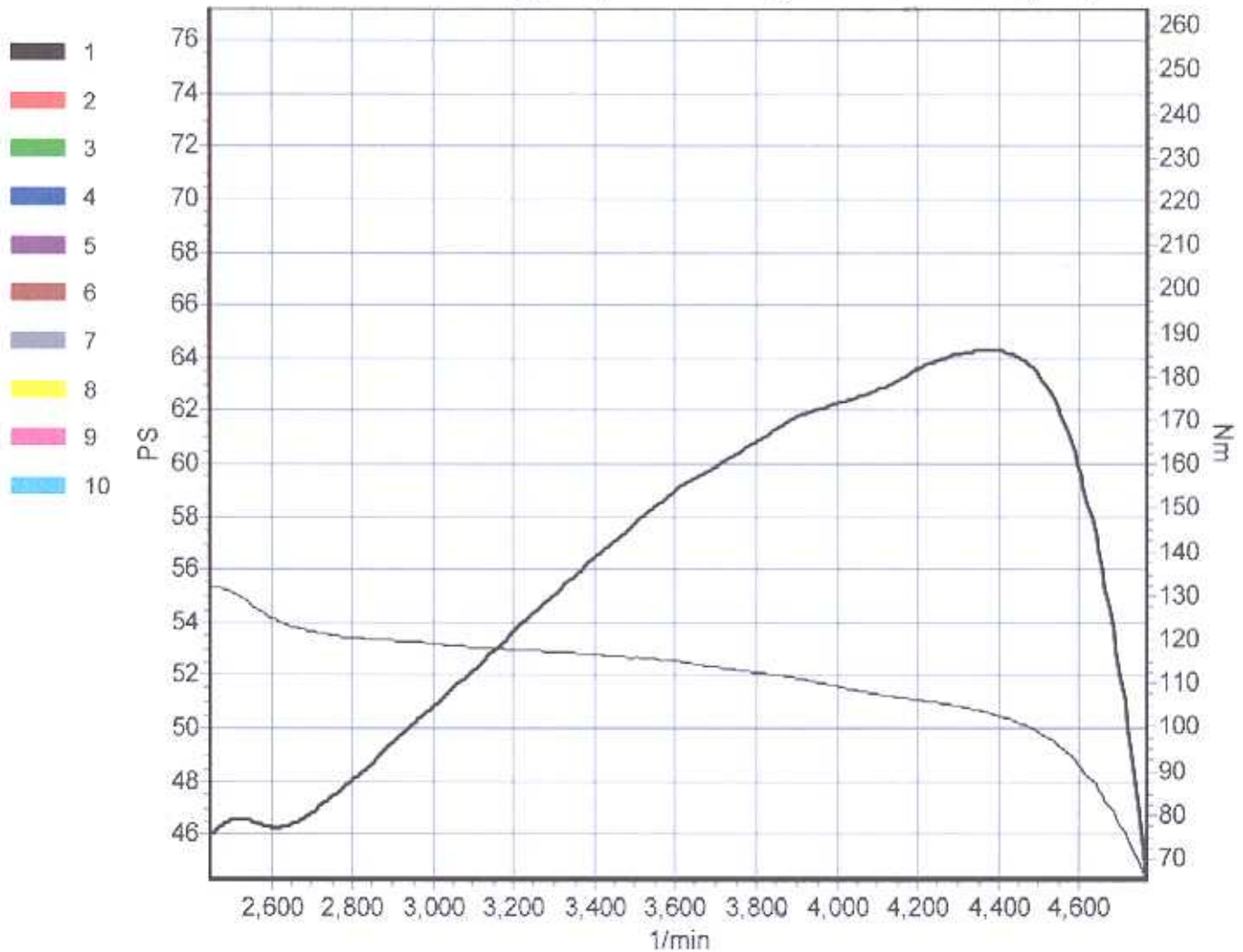
P-max Motorleistung (korr.) / Geschwindigkeit / Drehmoment (korr.)
